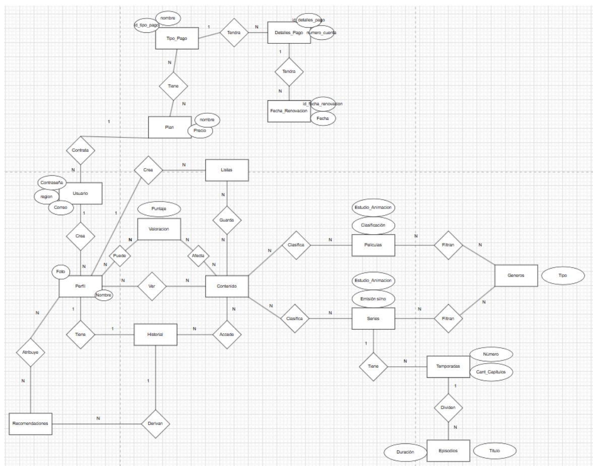
Modelo Entidad - Relacion hecho en draw.io
